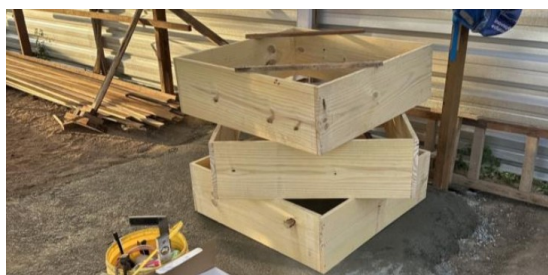
Figura 5. Fabricação de formas para sapatas.
