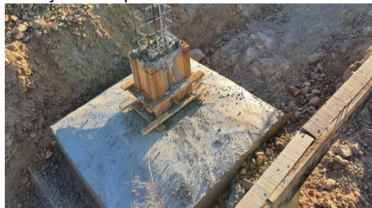
Figura 10. Montagem de forma, armação e concretagem de arranque de pilar.
