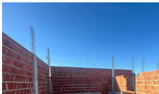
Figura 2. Montagem de armação de pilar.
