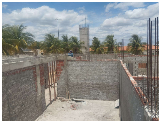
Figura 8. Aplicação de lastro de concreto magro em áreas de piso.
