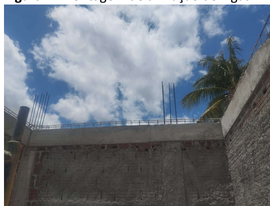
Figura 2. Montagem de armação de vigas.
